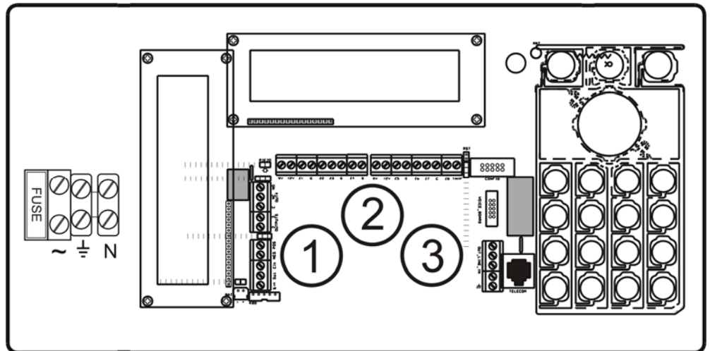
Fig. 2 Διάγραμμα Συνδέσεων IC60 compact
